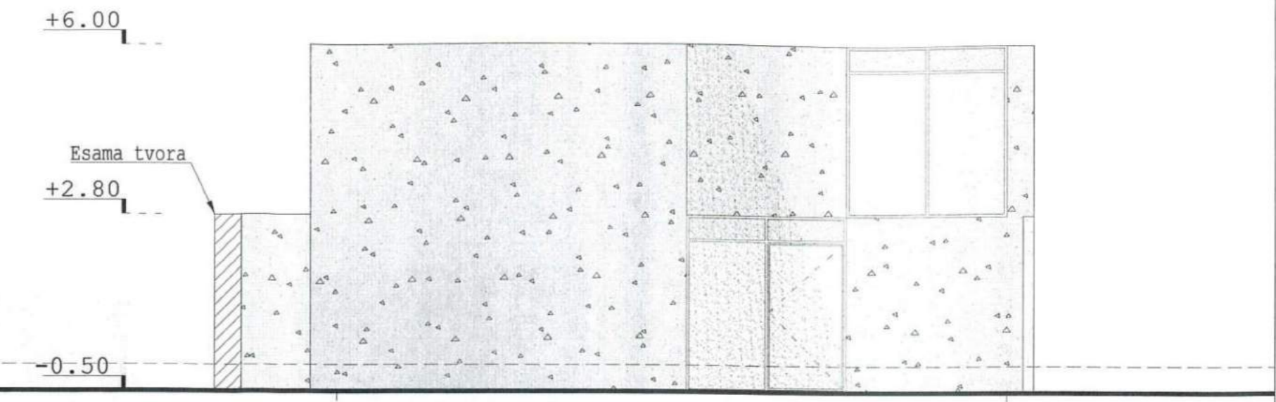
FASADAS TARP AŠIŲ Y1-Y3 M 1:100
