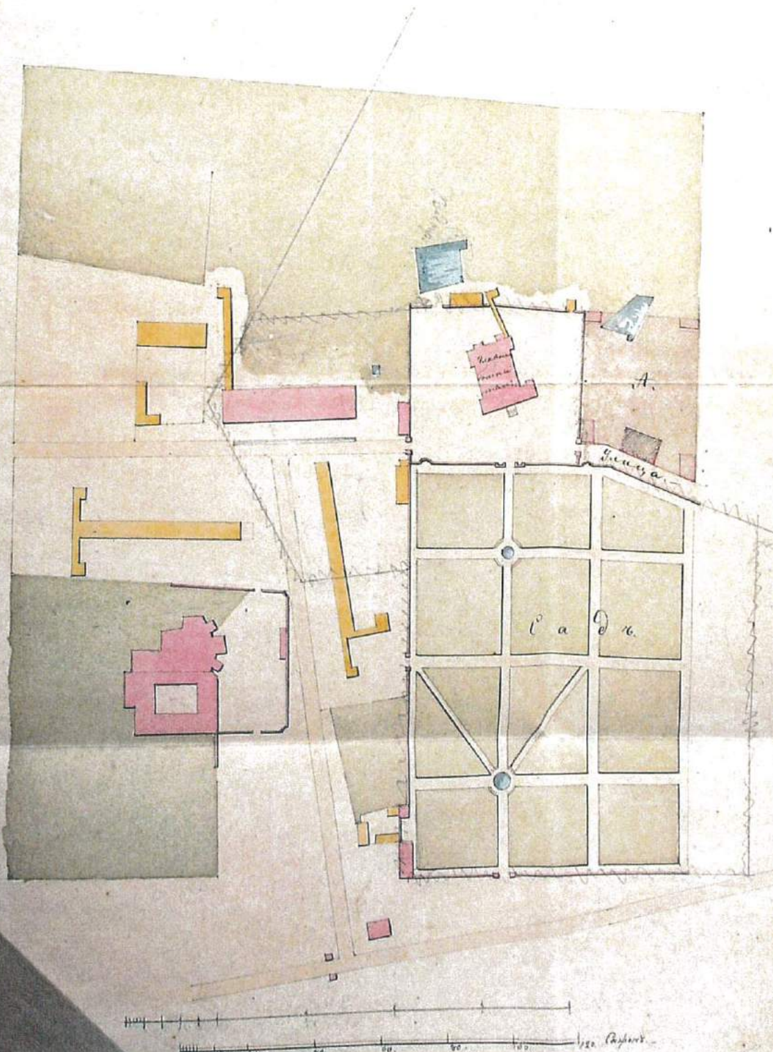
1840 m. geometrinis planas su numatomo statyti pastato vieta. Iš RACEVIČIENĖ, A.; BALIULYTĖ, I. Sapiegų rezidencijos, trinitorių vienuolyno ir ligoninės statinių komplekso teritorija. Užstatymo istorinė raida. VĮ „Lietuvos paminklai“ archyvas.
