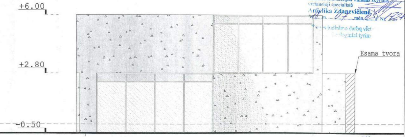
FASADAS TARP AŠIŲ Y3-Y1 M 1:100
